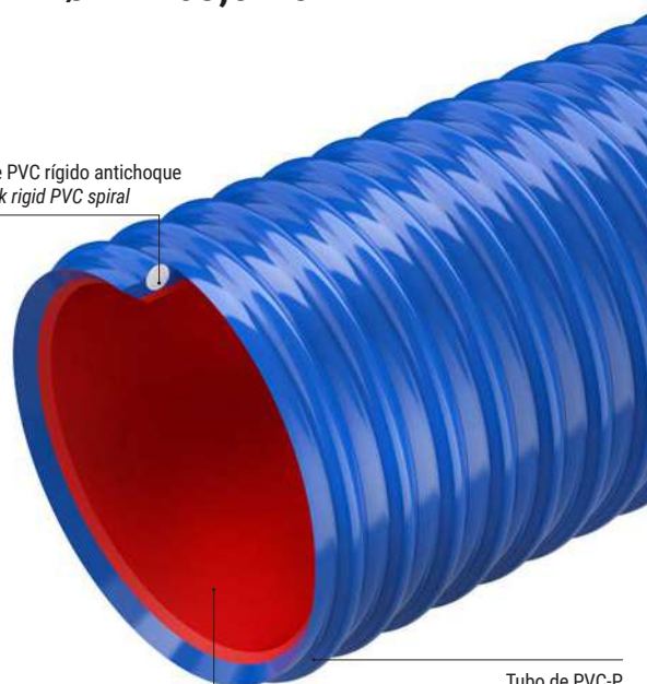
Capa inferior de TPU antiabrasivo Antiabrasive TPU liner
